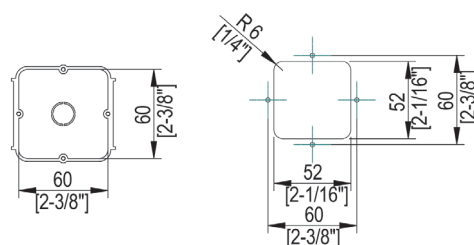
XS4 2.0 Wandler mit kapazitivem Tastenfeld
